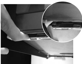
2. Auf die Klemmen drücken. Diese müssen in der gezeigten Position verbleiben.
